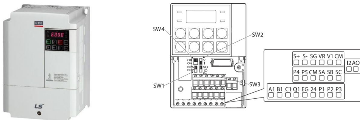
Fig. 1 Variador S100 y bornera de conexión
